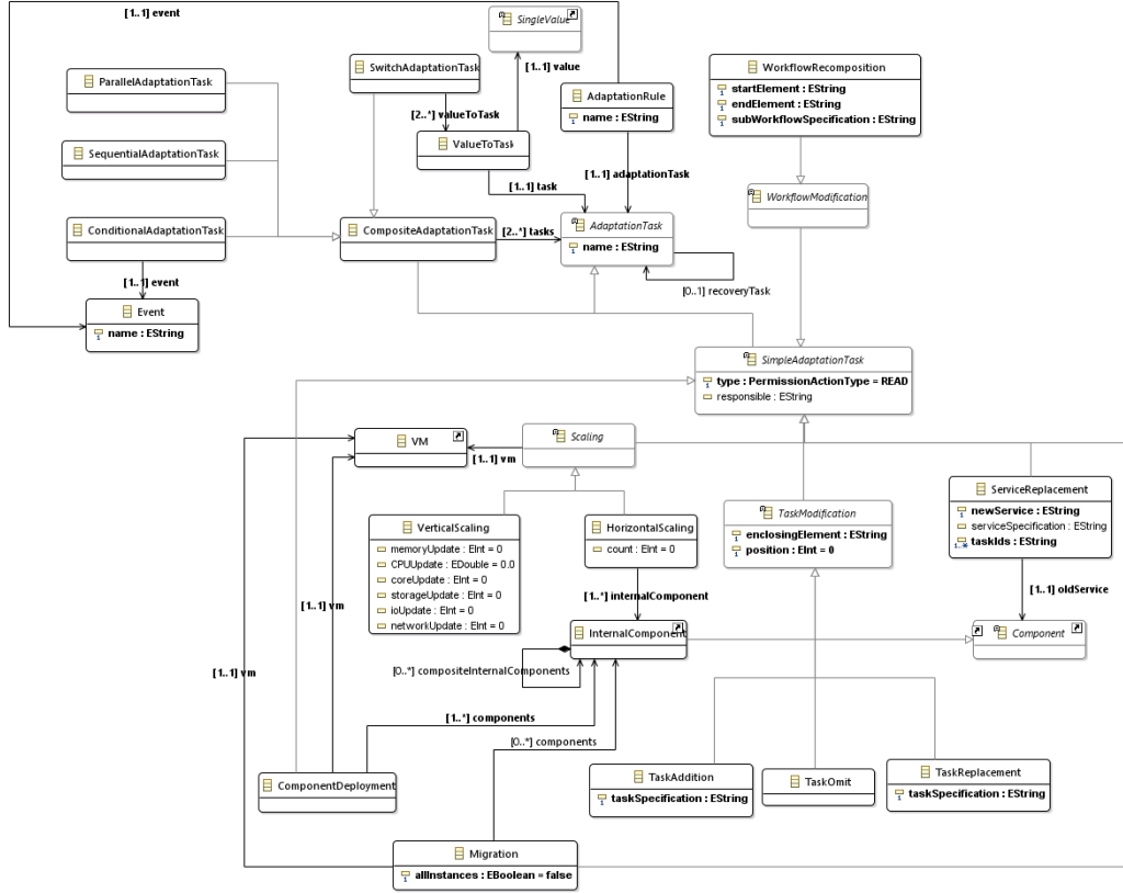
Fig. 2. The new SRL meta-model
